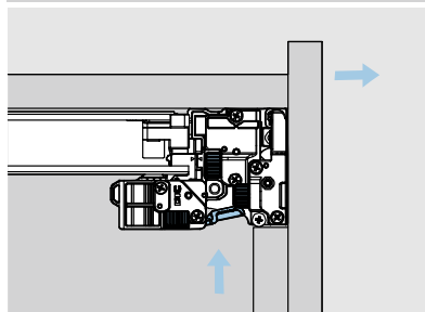
Pritisnite polugu na spojnici da biste izvukli fioku
