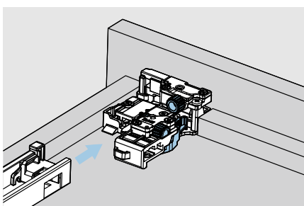
Montirati spojnicu šrafovim sa donje strane
