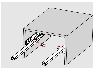
Montirati klizač na stranice korpusa
