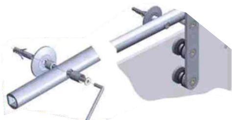
Prikaz montaže stopera i montiranja šine na zid
