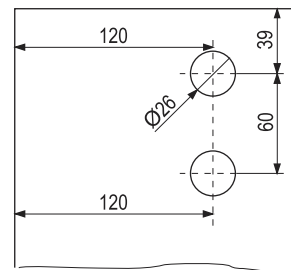
Dimenzije za pripremu (bušenje) stakla
