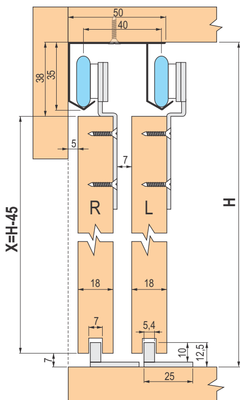
Al gornja dvokanalna šina SKM 38
