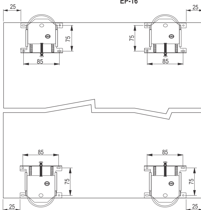
set metal 1610 Metalni mehanizam EP-16
