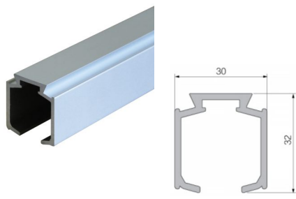
PVD TN gornja šina AL SM
