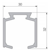
PVD TN gornja šina AL SM
