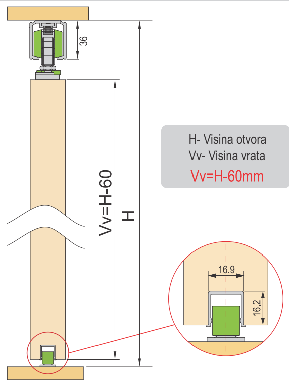
PVD TN gornja šina AL SM
