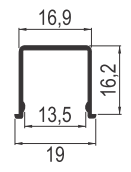
PVD OP-8 donja vodica AL
