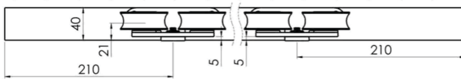
Prikaz pozicioniranja gornjih mehanizama na vrata (ispunu)
