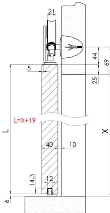
Prikaz montiranja šine bez distancera
