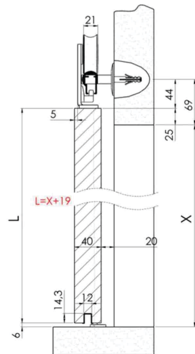
Prikaz montiranja šine sa distancerom
