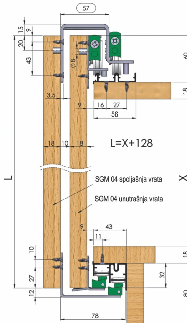
Prikaz montaže unutrašnjeg mehanizma
