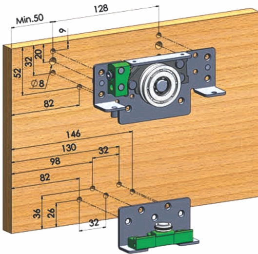
Prikaz montaže unutrašnjeg mehanizma
