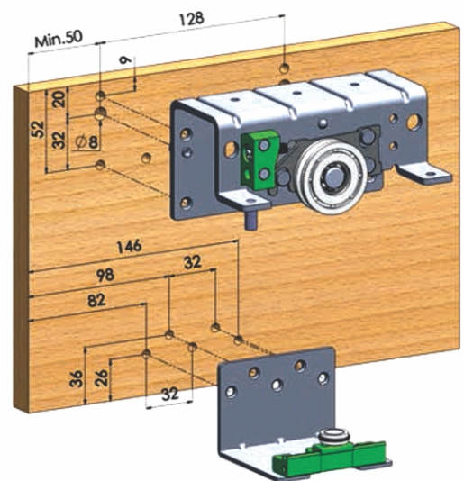
Prikaz montaže spoljašnjeg mehanizma
