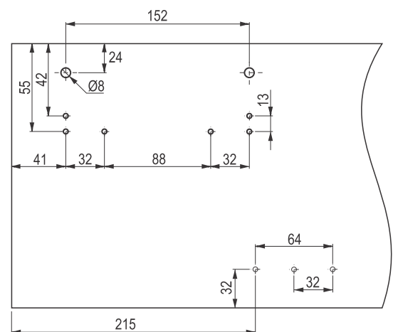
Postavljanje unutrašnjeg mehanizma
