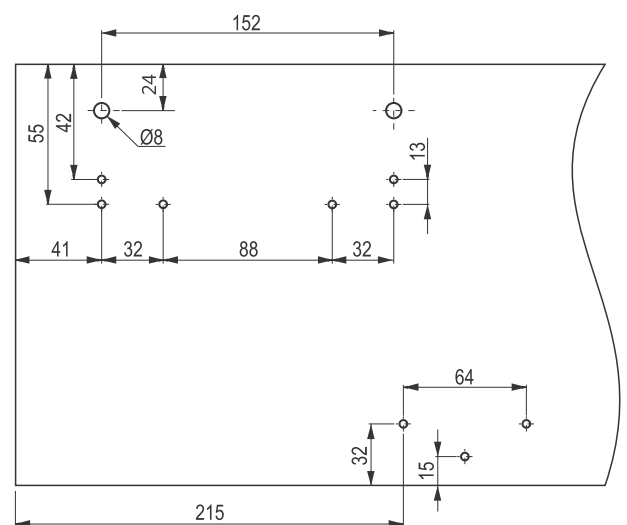
Postavljanje spoljašnjeg mehanizma
