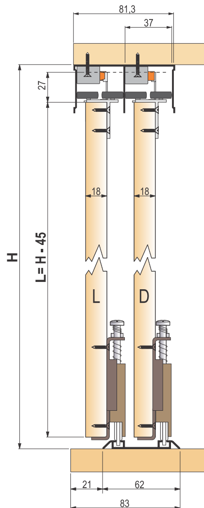
Izračunavanje visine vrata kada se koristi EP set usporivača do 60kg
