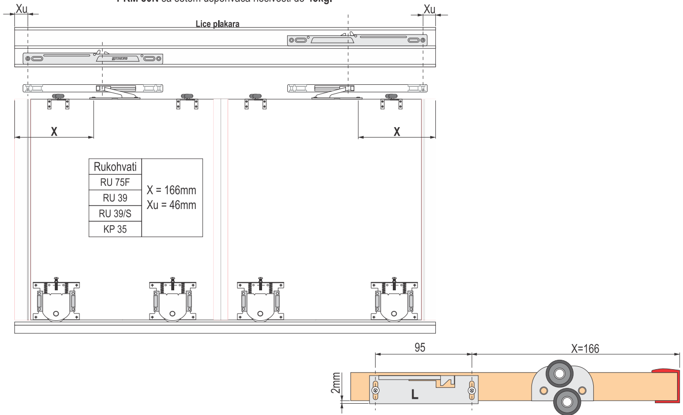
PKM 80N sa setom usporivača nosivosti do 45kg.
