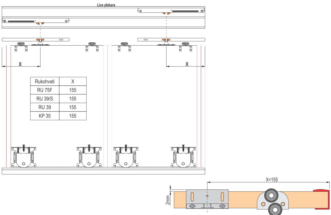
PKM 80N sa setom usporivača nosivosti do 60kg.
