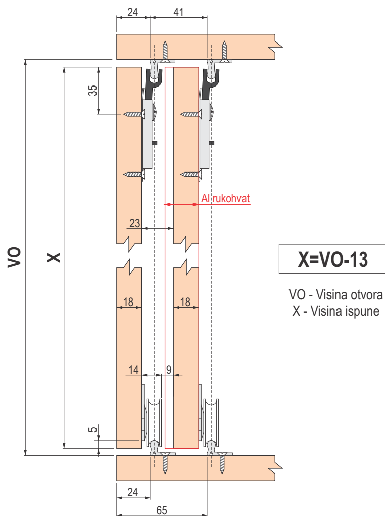
Šema montaže mehanizma sa ispunom debljine 18 mm
