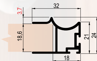
SM - 70 AL UKRUTNI RUKOHVAT
