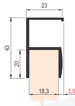
SM - 39 S AL RUKOHVAT
