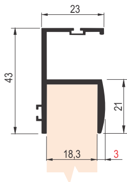
SM - 39 AL RUKOHVAT
