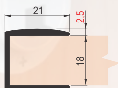
SM - 35 AL UKRUTNI RUKOHVAT
