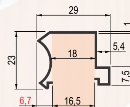
SM - 16 AL UKRUTNI RUKOHVAT
