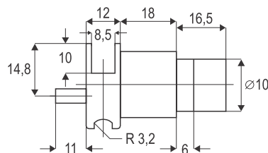
Tehnički crteži SS SI 2010 bravice
