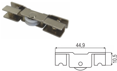
SS SI 2010 met.mehanizam
