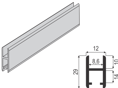
SS SI 2010 donja vodica 2m AL SM
