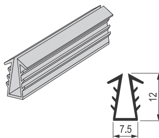
SS SI 2010 PVC za donju vodicu
