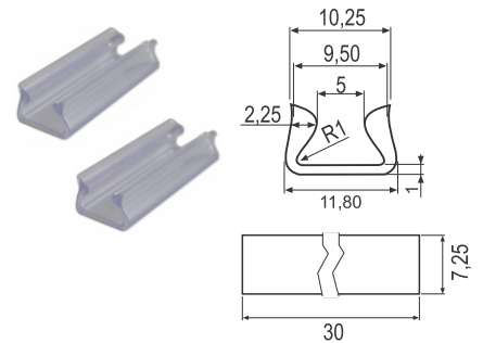
SS SI 2010 PVC za gornju vodicu
