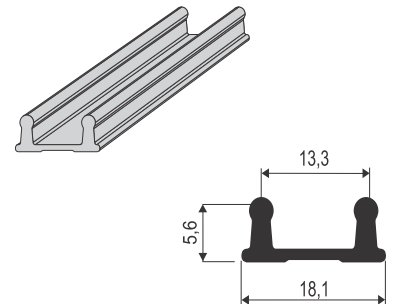
SS SI 2010 donja šina 2m AL SM
