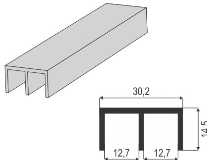
SS SI 2010 gornja šina 2m AL SM
