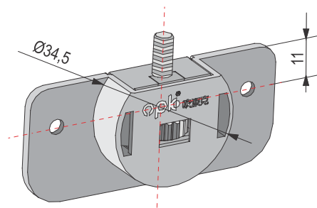
PVC gornji mehanizam ukopavajući
