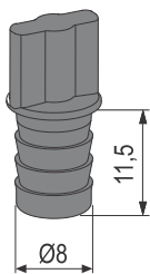
PVC usmerivač pravca ukopavajući
